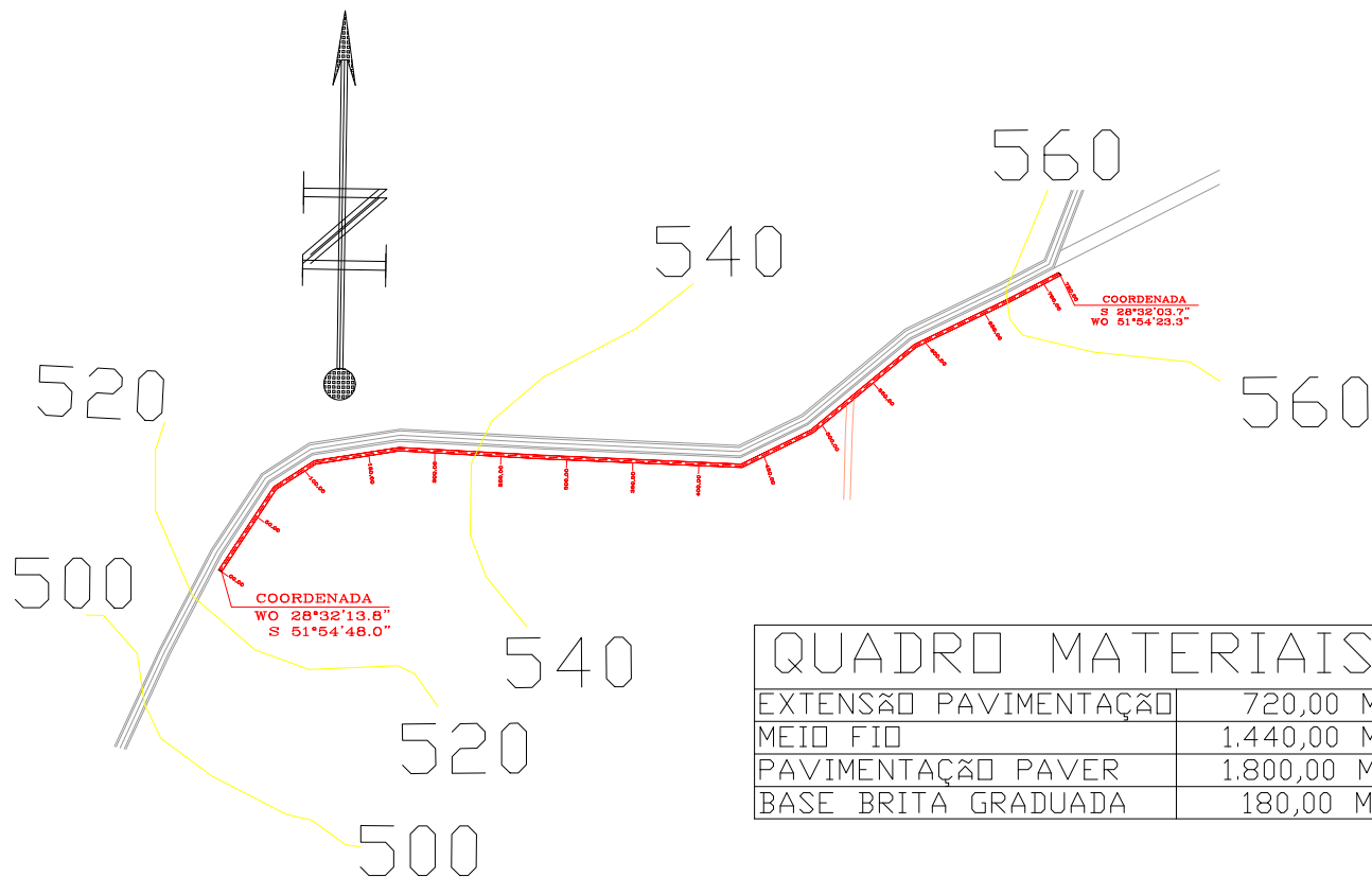
LEVANTAMENTO PLANIALTIMÉTRICO ESC.: 1: 2000
