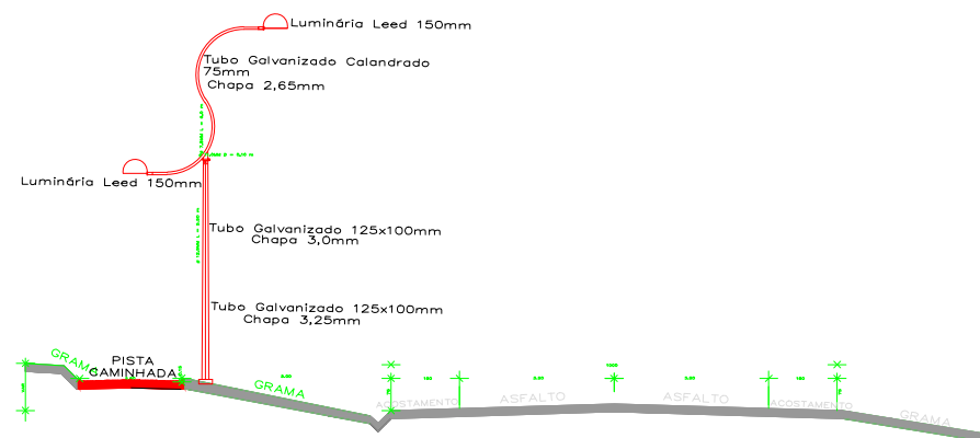
CORTE TRANSVERSAL COM POSTES DE ILUMINAÇÃO PÚBLICA
