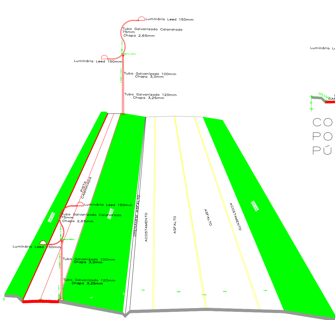
PERFIL PISTA DE CAMINHADA; POSTES DE ILUMINAÇÃO PÚBLICA
