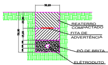
DETALHE DA VALA DOS ELETODUTOS ENTERRADOS ESC. S/N
