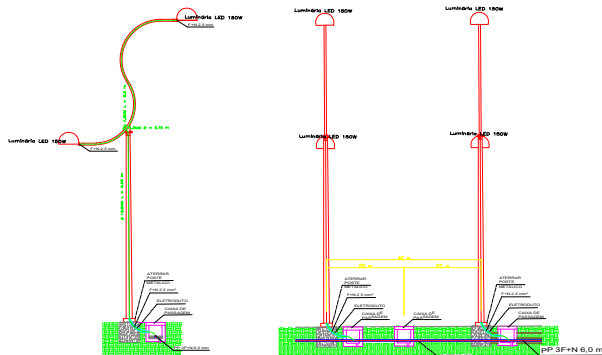
DETALHE TRANSVERSAL INSTALAÇÃO DOS POSTES E REDE ELÉTRICA ESC. S/N
